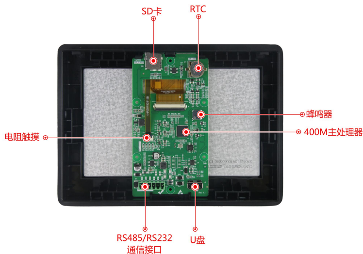
图 1-2 硬件配置图
